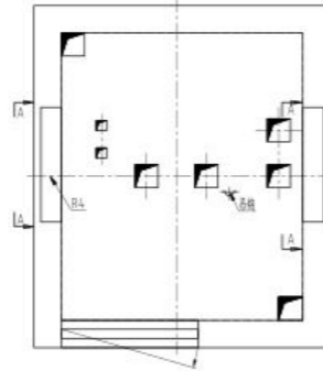
机房留孔图
