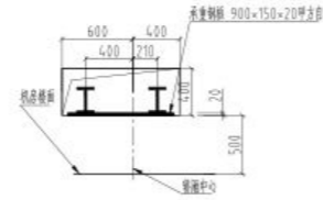
A-A承重孔
